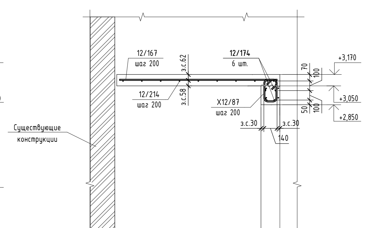
2-2 Армирование
