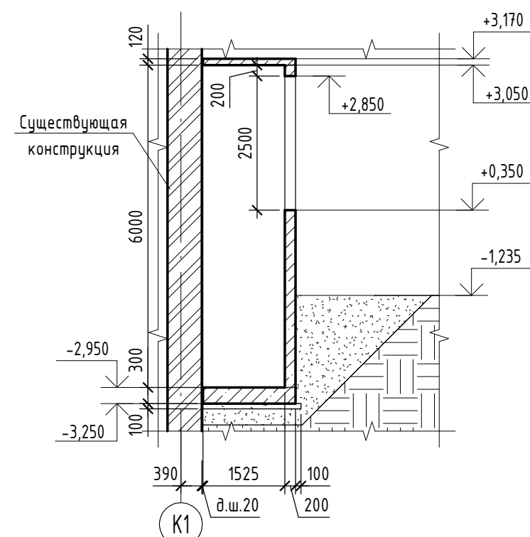
2-2 Опалубка
