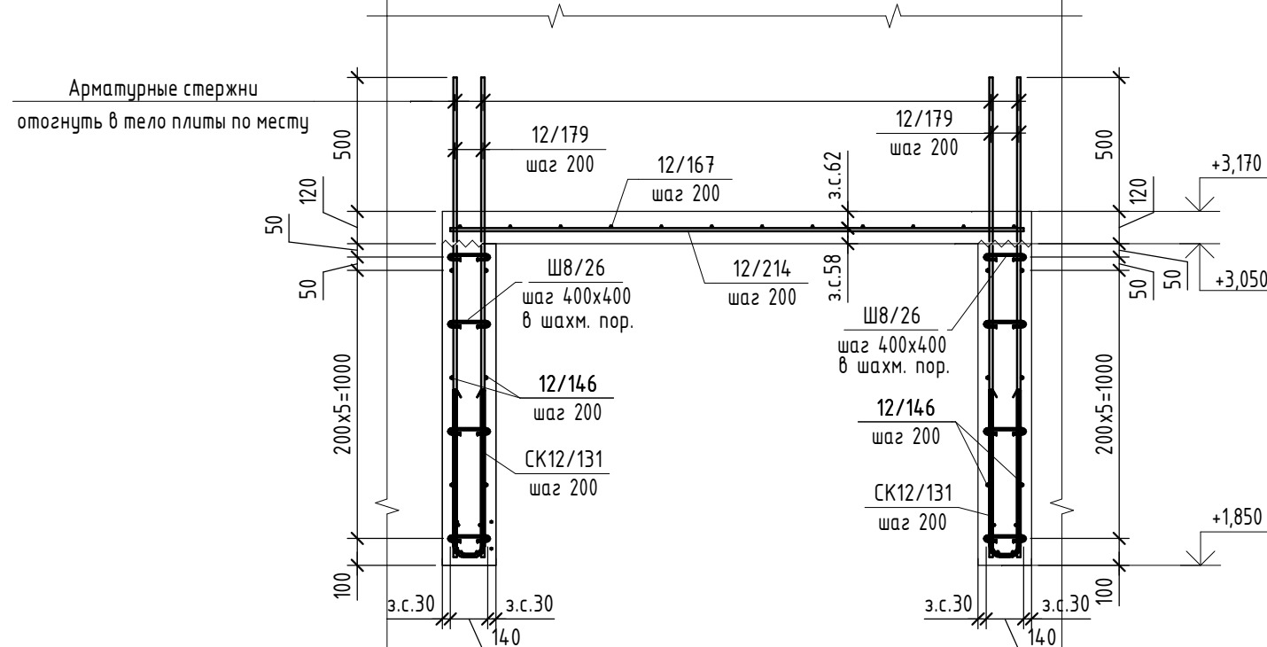
1-1 Армирование
